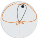
图 4 R310 2.4GHz 鲁拜 天线模式
